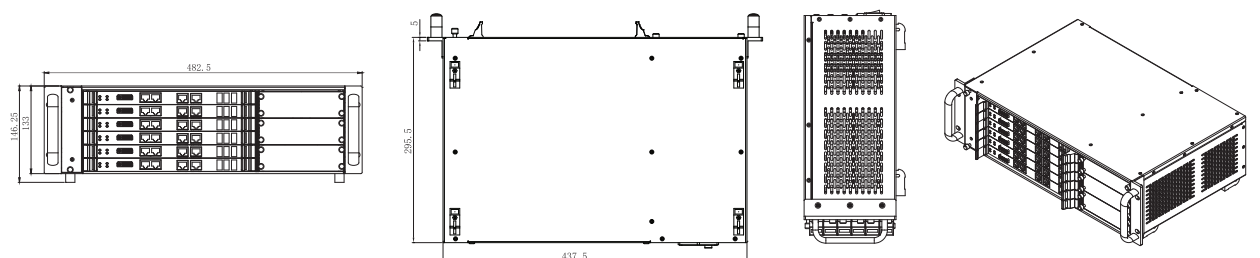
CPCIC-7606A 尺寸图
