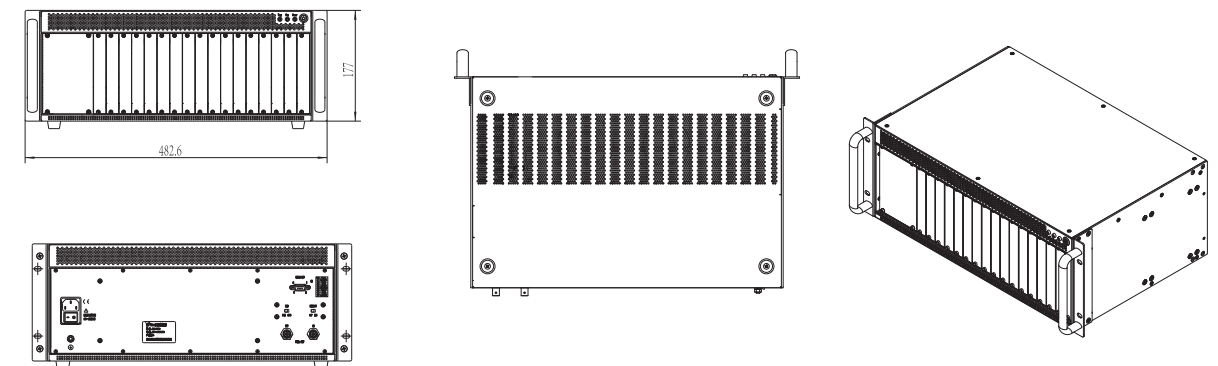
PXIC-7318C 尺寸图
