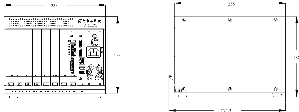
PXIC-7306 尺寸图
