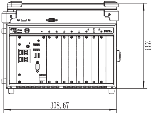
PXIeA-39525 尺寸图
