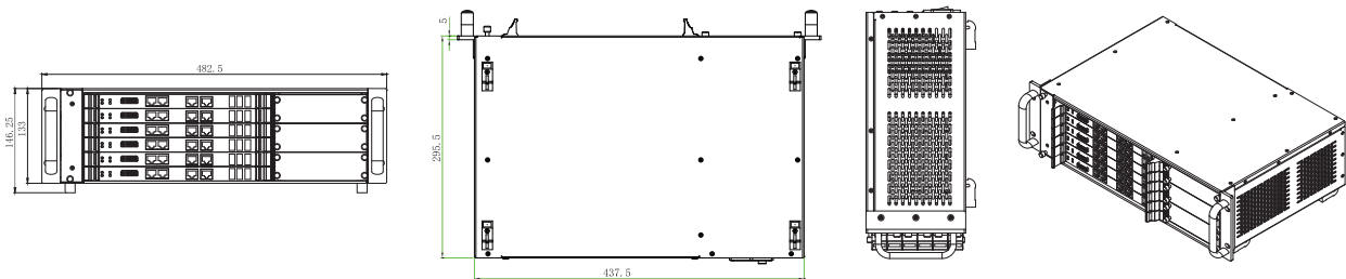
CPCIC-7606 尺寸图
