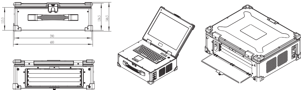
CPCIA-64513 尺寸图
